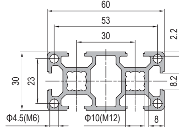
30x60 6 slots
