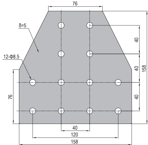
PG40-8080-02
