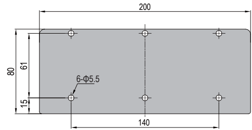
Conduit Cap-80x200
