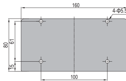
Conduit Cap-80x160
