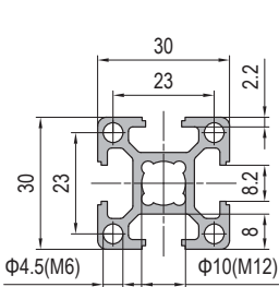
30x30 4 slots
