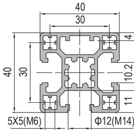
40x40 3 slots
