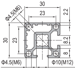
30x30 4 slots
