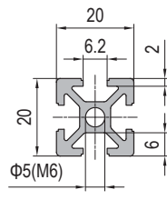
20x20 4 slots
