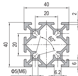
40x40 8 slots
