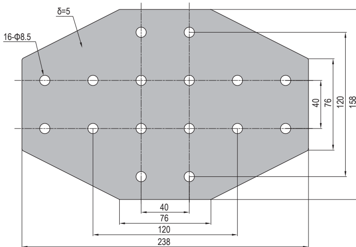
PG40-8080-03
