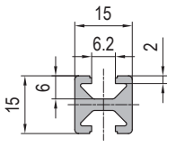
15x15 2 slots
