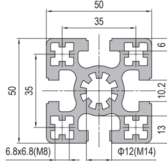
50x50 4 slots
