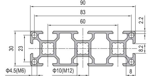
30x90 8 slots
