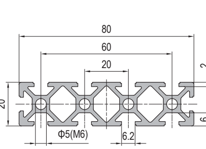
20x80 10 slots
